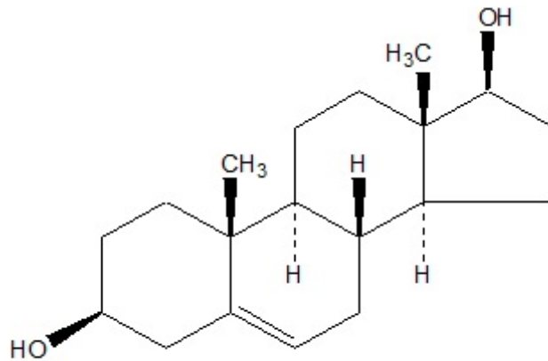
Androstenediol
